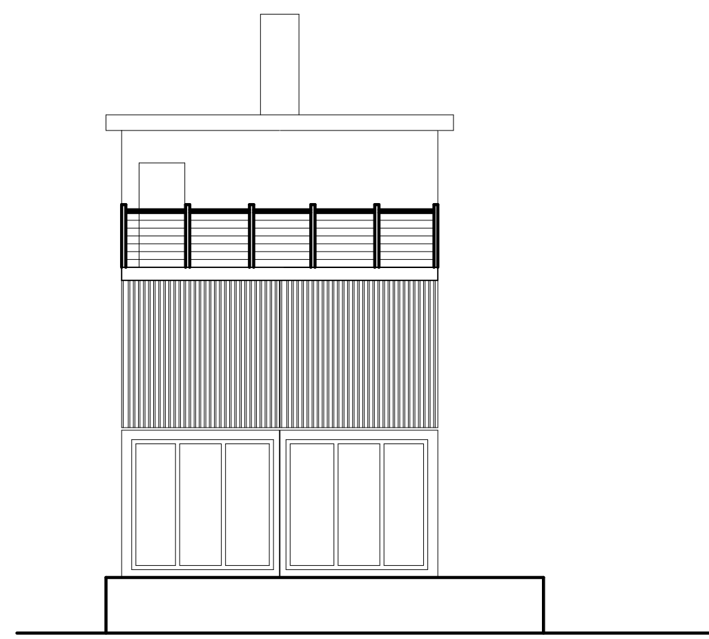
Ansicht Links
