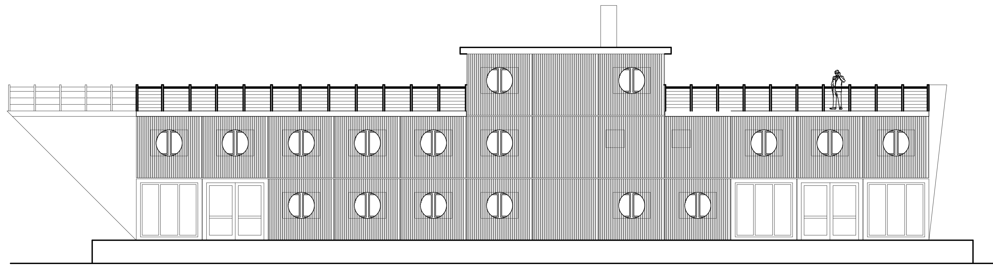
Ansicht Seeseite
